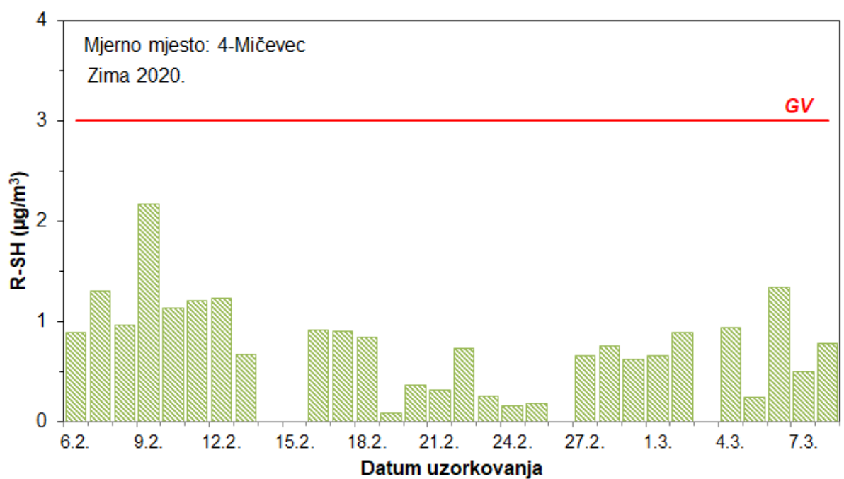
Slika 33 – Kretanje srednjih dnevnih koncentracija merkaptana na mjernoj postaji 4 – Mičevec tijekom zimskog razdoblja mjerenja
