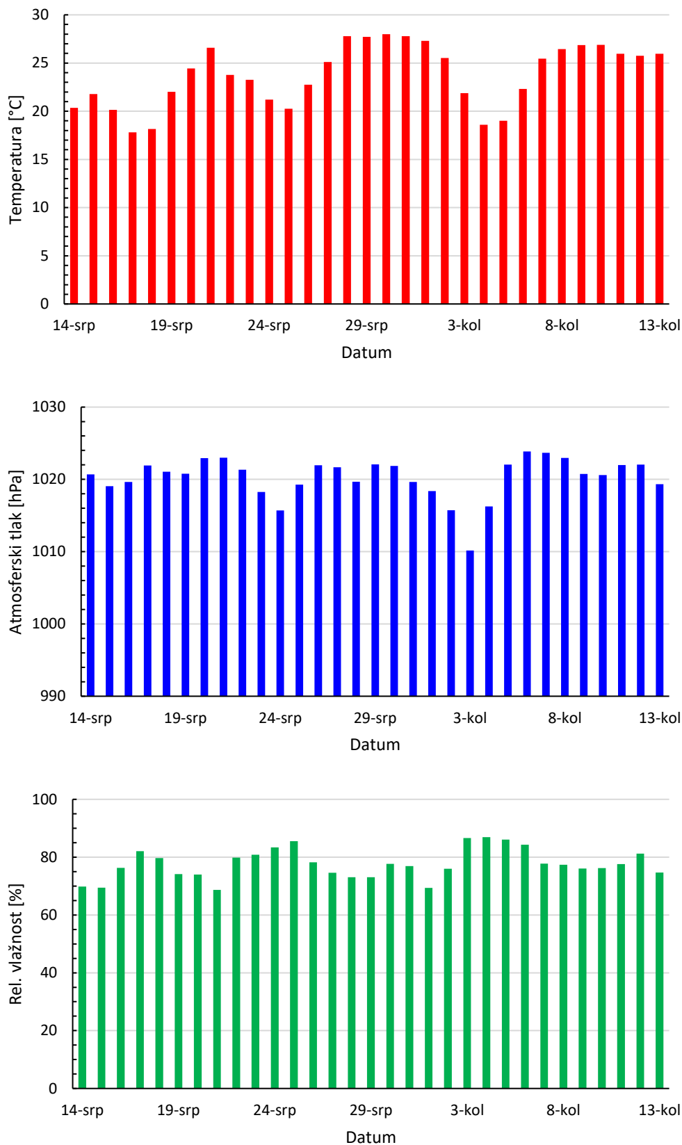
Slika 48 - Dnevni srednjaci temperature, tlaka i relativne vlažnosti na mjernoj postaji 1 –Biologija sjever određeni tijekom ljetnog razdoblja
